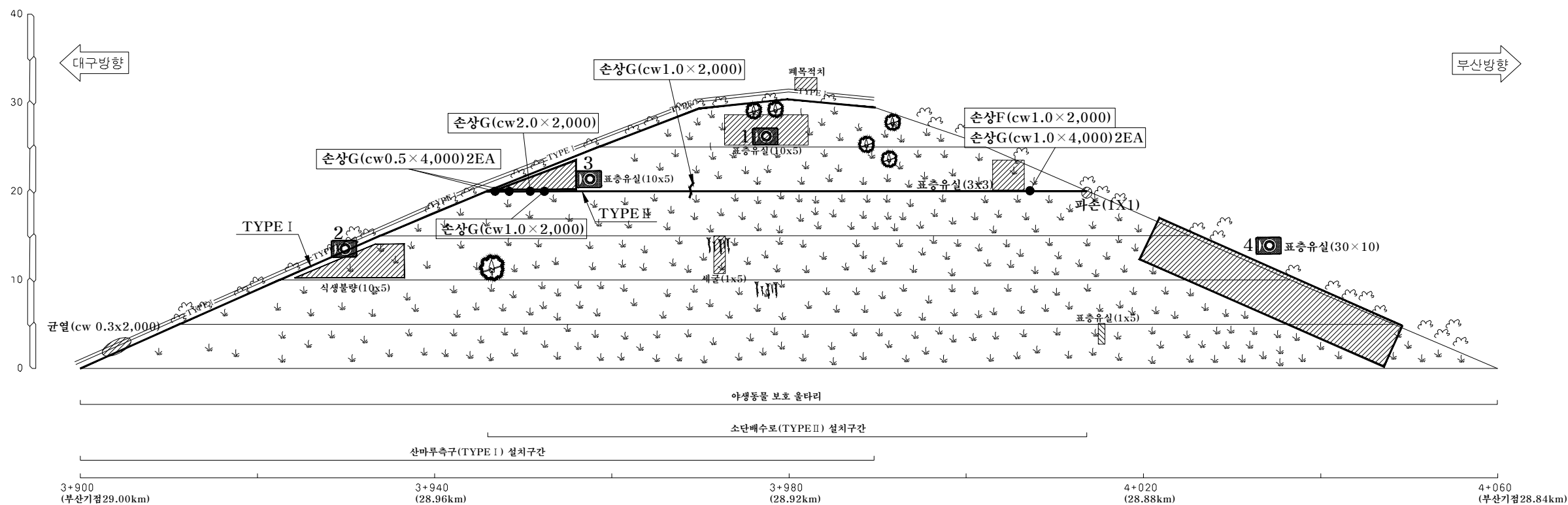
대구절토37/부산기점 28.84~29.00km (9공구 STA.3+900~4+060)
